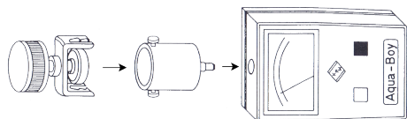
Raccordement avec électrode à godet
